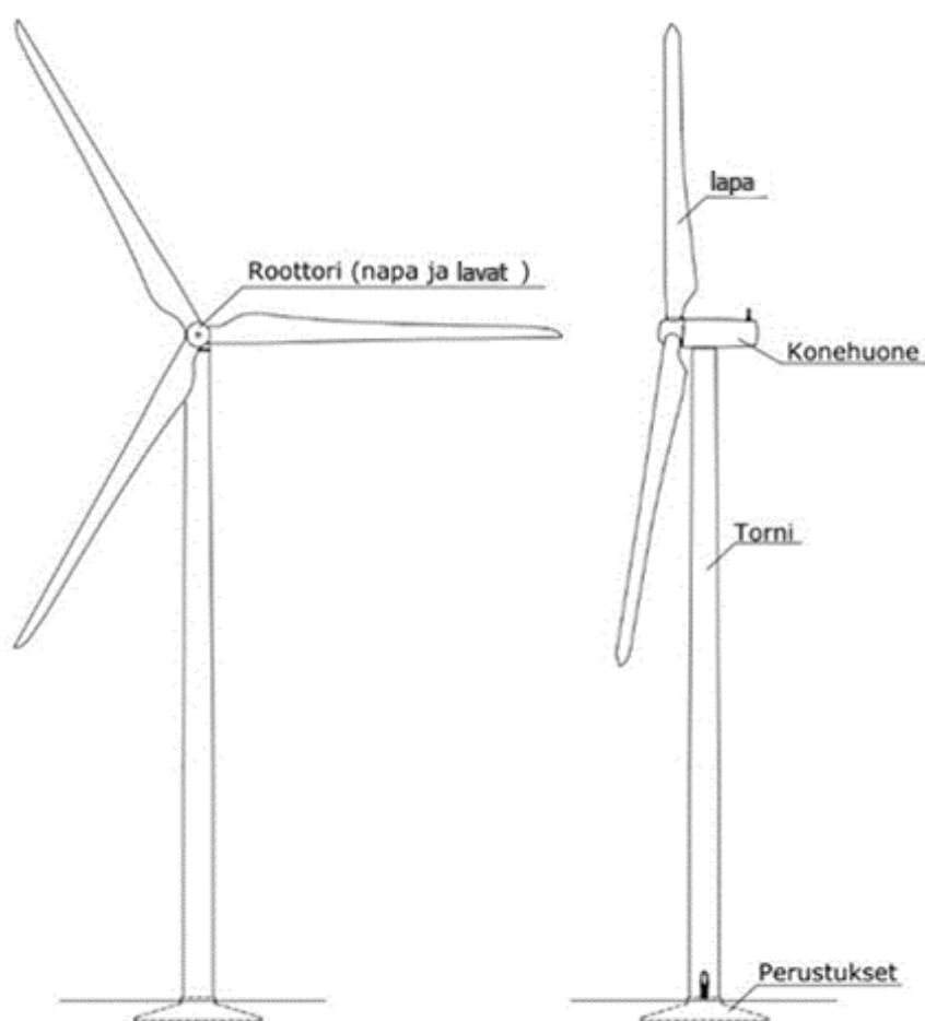
Kuva 3-1. Tuulivoimalan periaatekuva.
