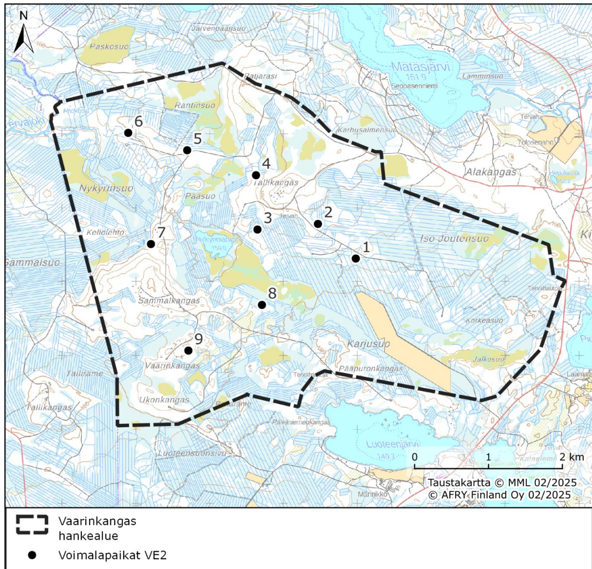
Kuva 2. Vaarinkankaan tuulivoimahankkeen voimalapaikat vaihtoehdossa VE2.
