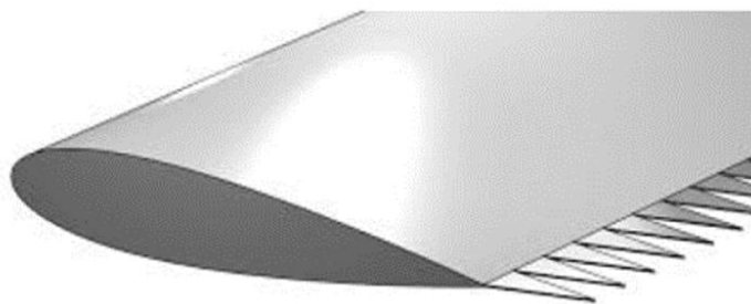
Kuva 3-13. Havainnollistus tuulivoimalan lavan jättöreunan sahalaoidituksesta (Martinez et al., 2019).
