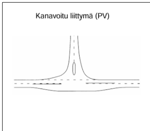
Kuva 14. Kanavoitu liittymä
