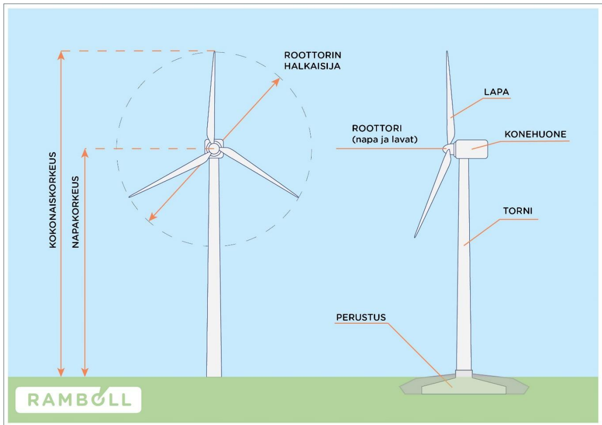
Kuva 6-1 Tuulivoimalan periaatekuva.
