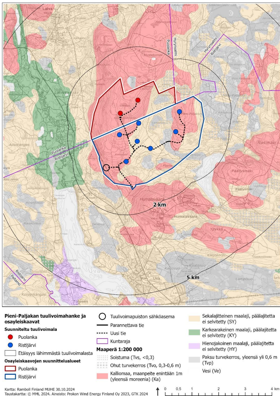
Kuva 4-3. Suunnittelualueen maaperä.
