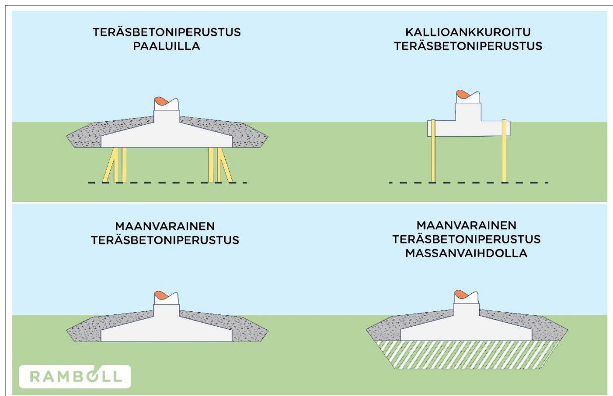
Kuva 6-2. Tuulivoimaloiden perustamistekniikoita.
