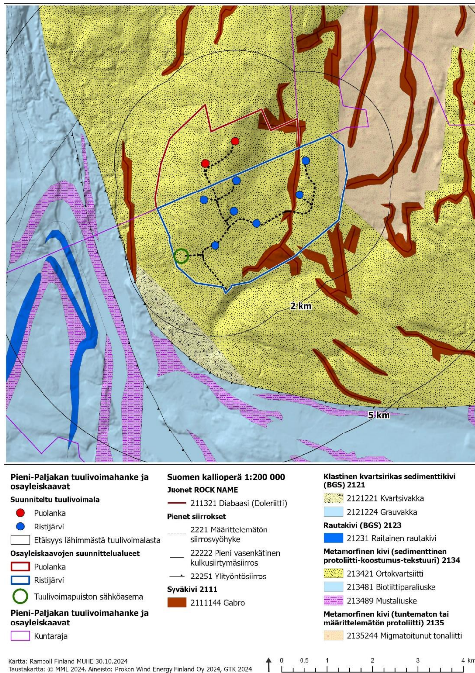
Kuva 4-4. Suunnittelalueen kallioperä.
