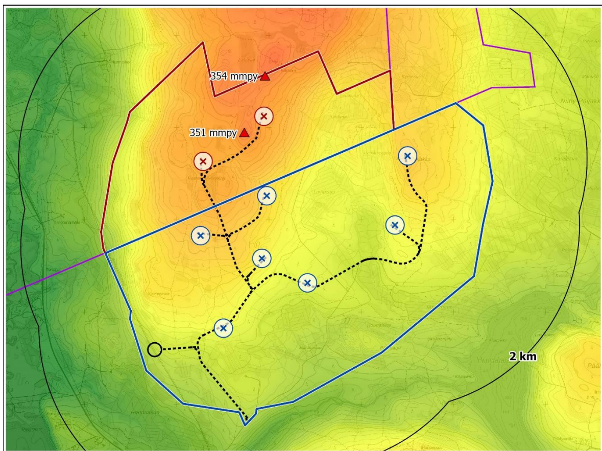
Kuva 4-2. Suunnittelualueen korkeusmalli.
