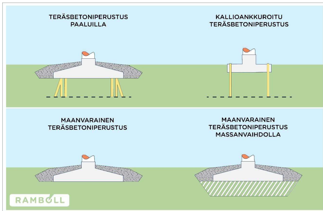
Kuva 6-2. Tuulivoimaloiden perustamistekniikoita.
