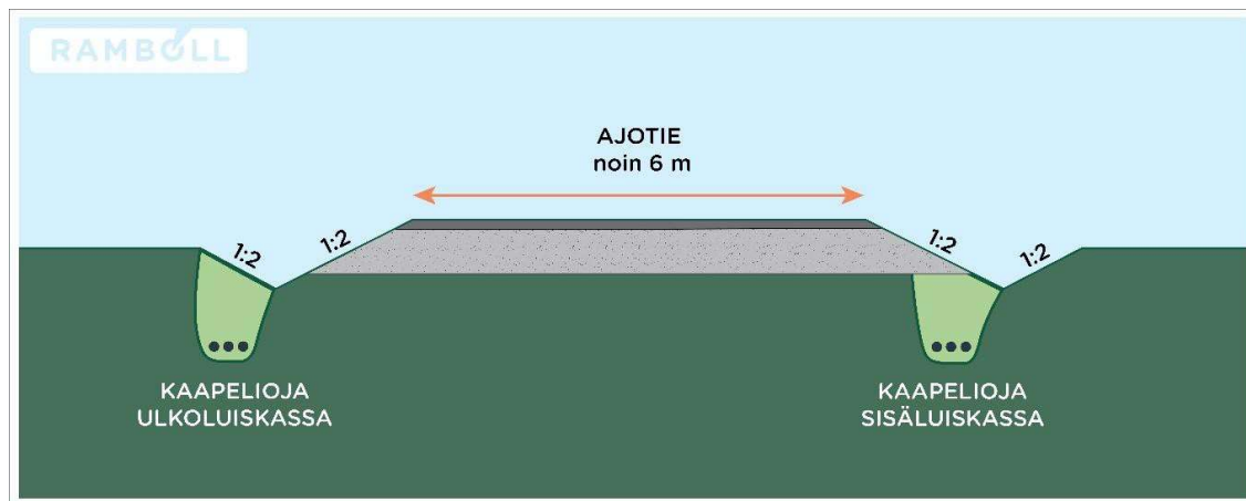
Kuva 6-3. Periaatekuva huoltotien rakenteesta.
