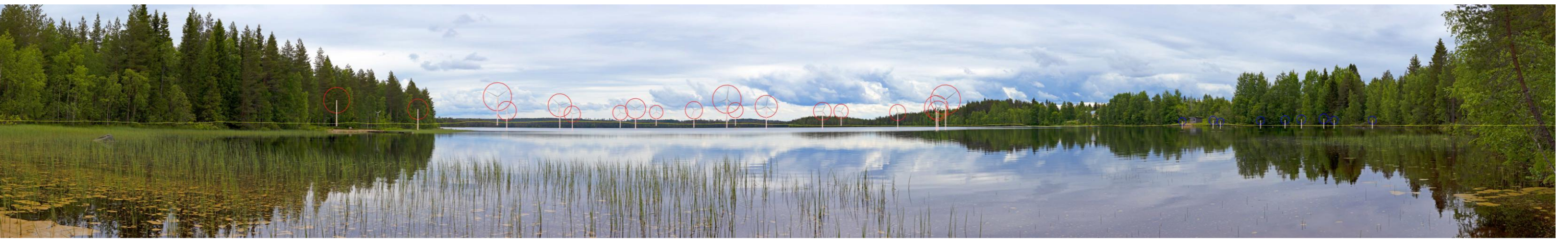
Kuva 37. Havainnekuvaluonnos kuvauspisteestä 10 hankevaihtoehdossa 1 (VE1), Isojärven ranta (Hautala). Etäisyys lähimpään Koirakankaan ja Hirvivaara-Murtiovaaran voimalaan on noin 3,8 kilometriä. Koirakankaan voimalat on korostettu sinisellä roottoriympyrällä ja Hirvivaara-Murtiovaaran punaisella roottoriympyrällä.
